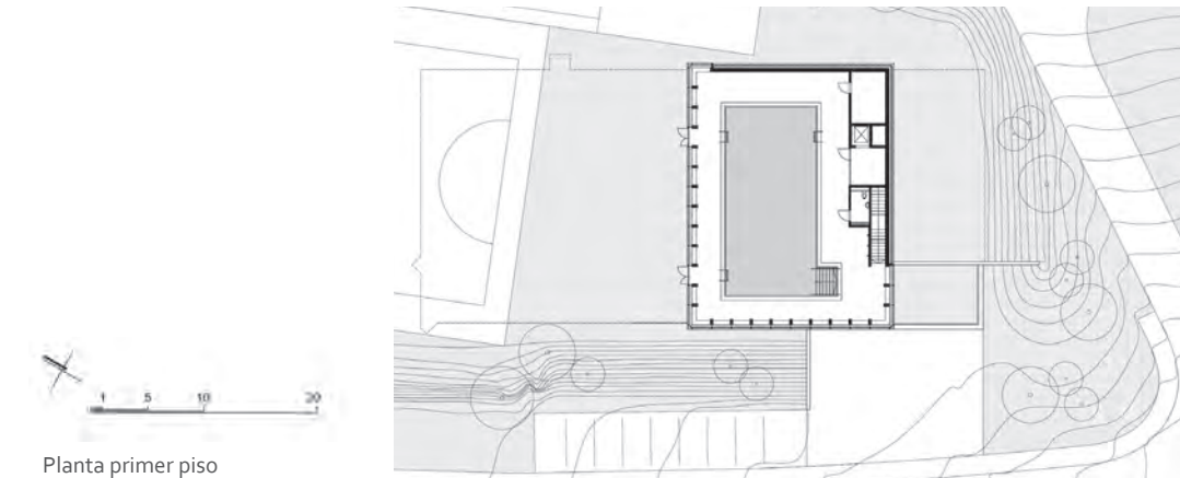
Planta primer piso
