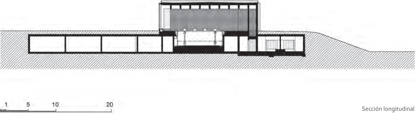
Sección longitudinal
