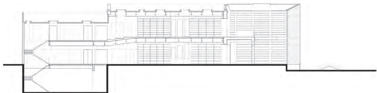
Sección logitudinal
