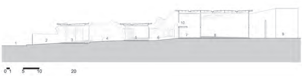
Corte longitudinal B-B
