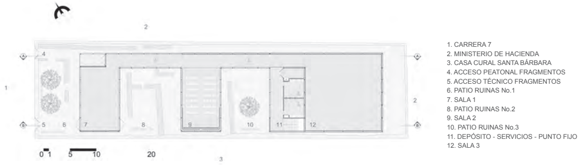
Planta primer piso
