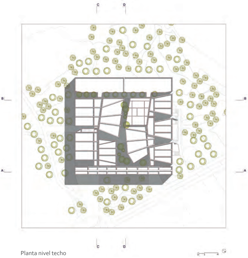
Planta nivel techo
