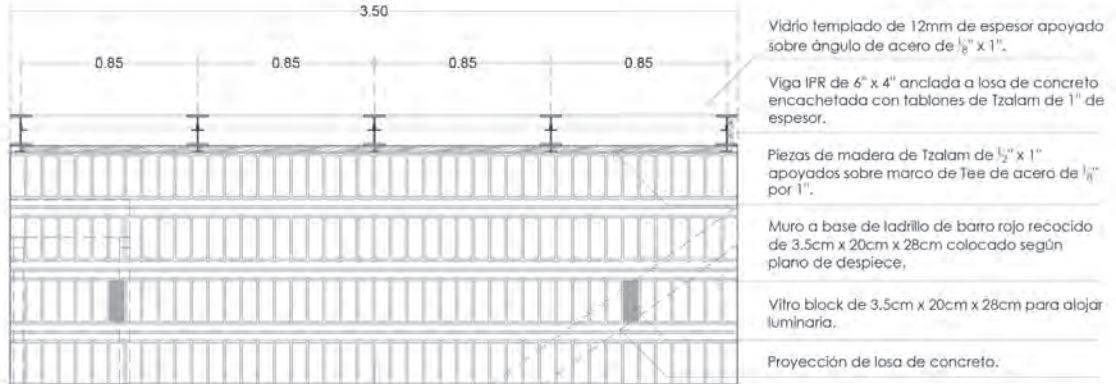
DETALLE CUBIERTA TERRAZA
