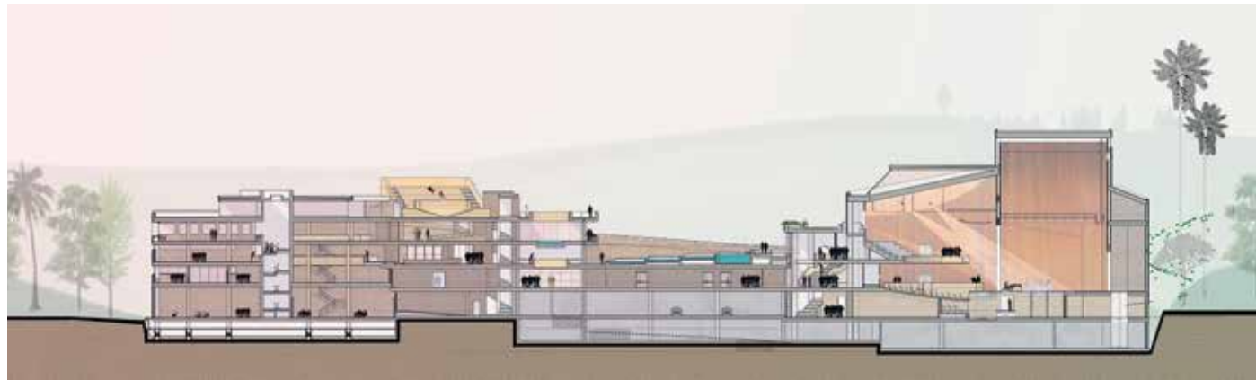
Sección longitudinal
