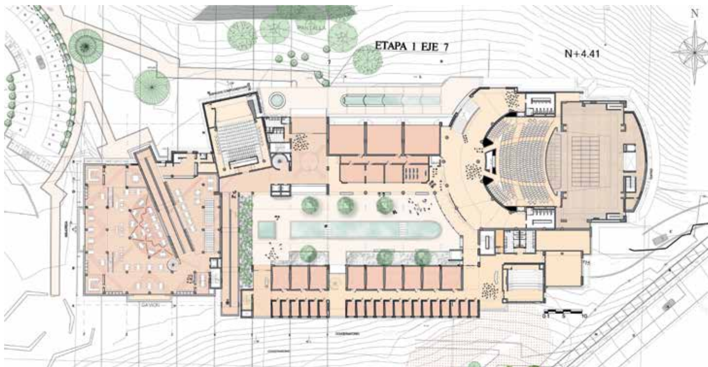
Planta general Nivel+4,41m.
