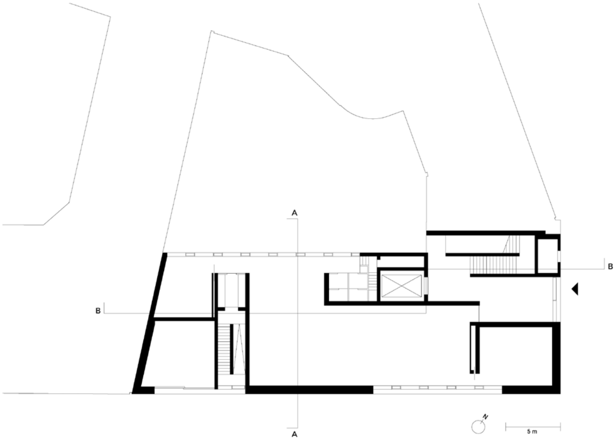
Planta Nivel 0
