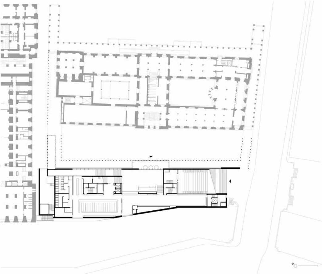
Planta Nivel 1 y Mezanine
