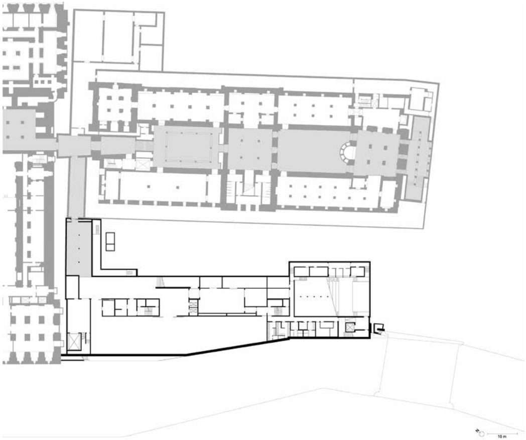
Planta Nivel 0
