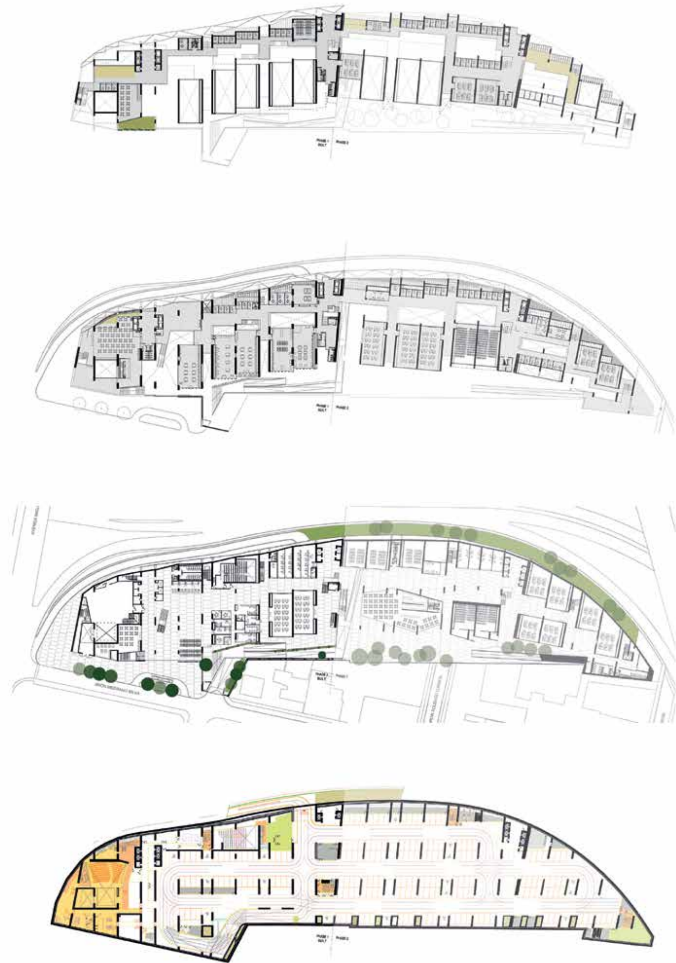
Plantas (de abajo hacia arriba: Nivel -1, Nivel 0, Nivel 1, Nivel 2)
