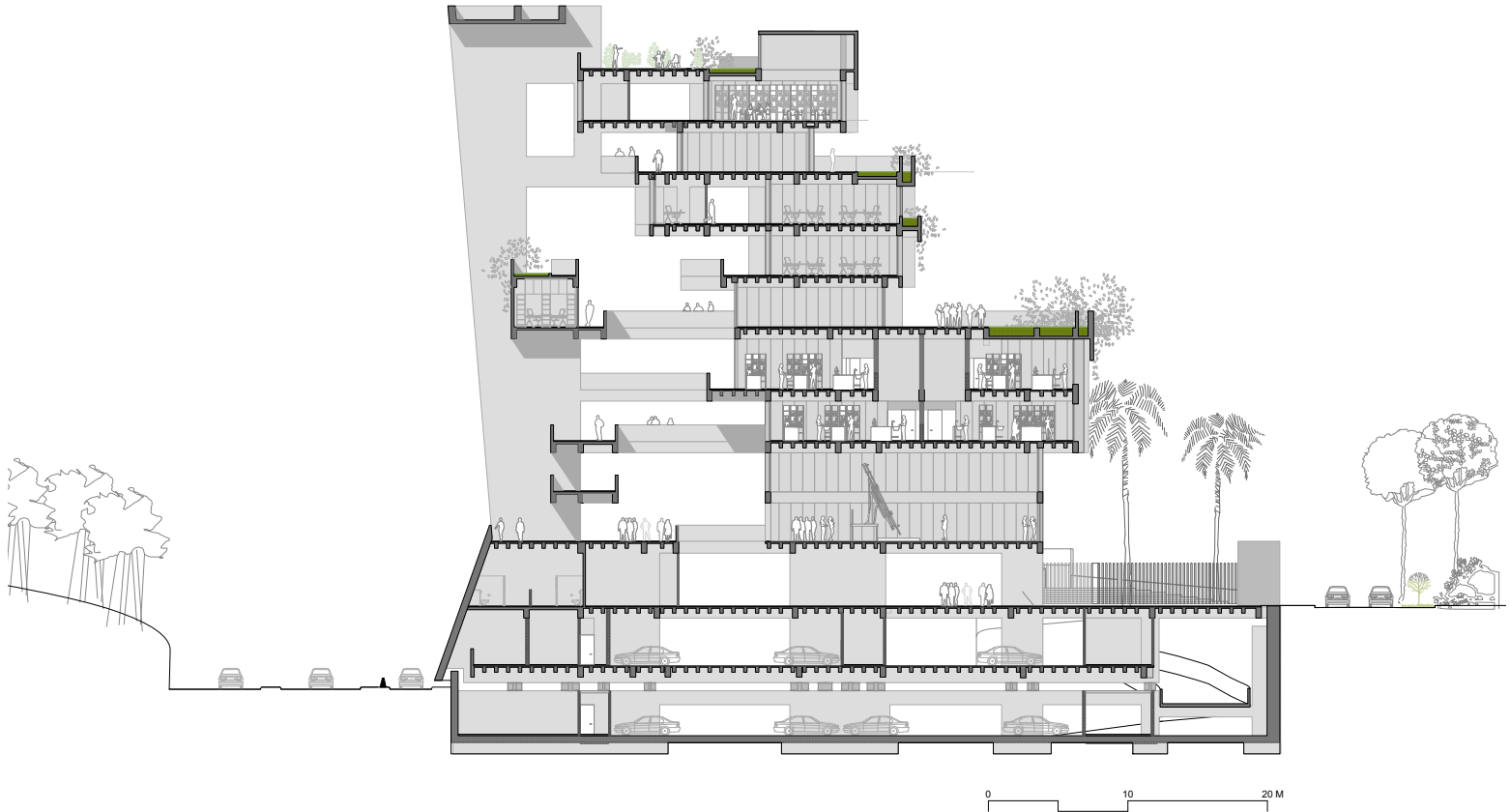
Sección transversal
