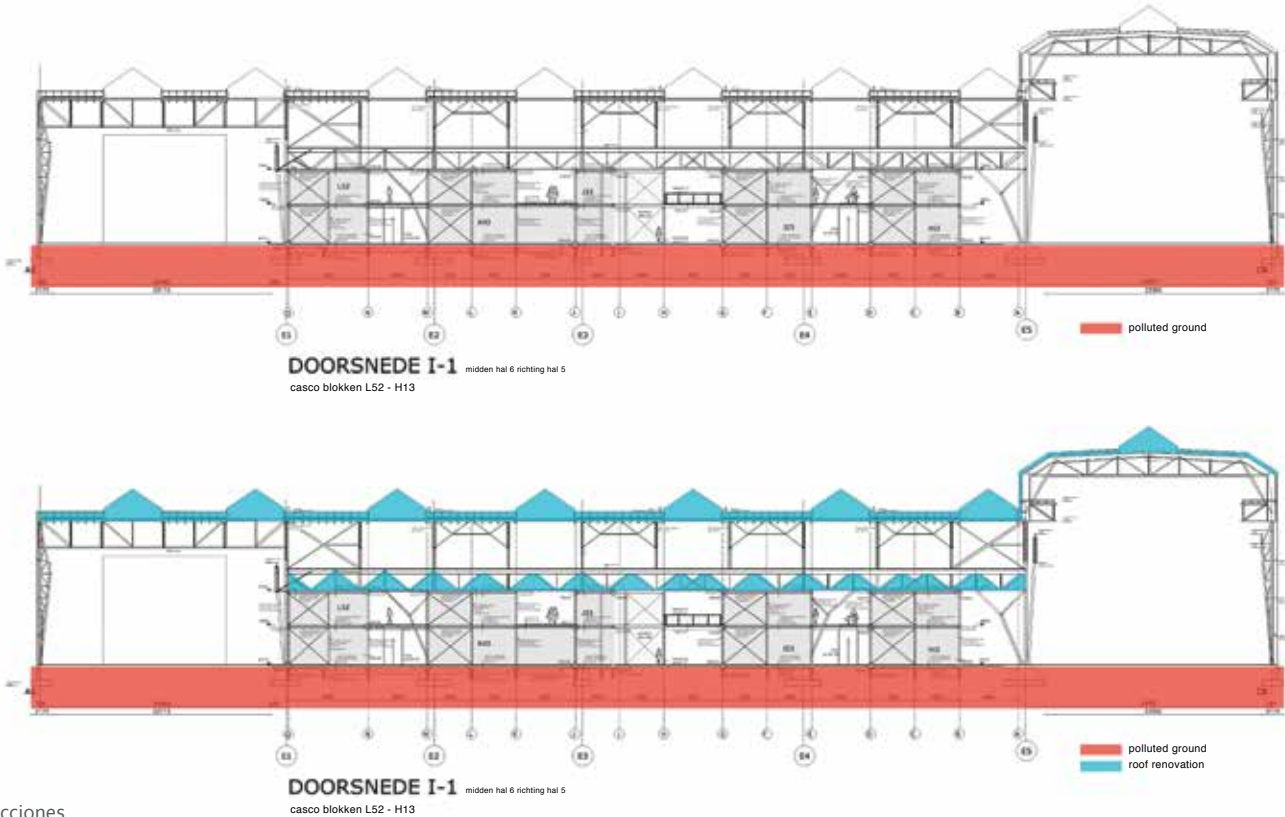
Sections / Secciones
