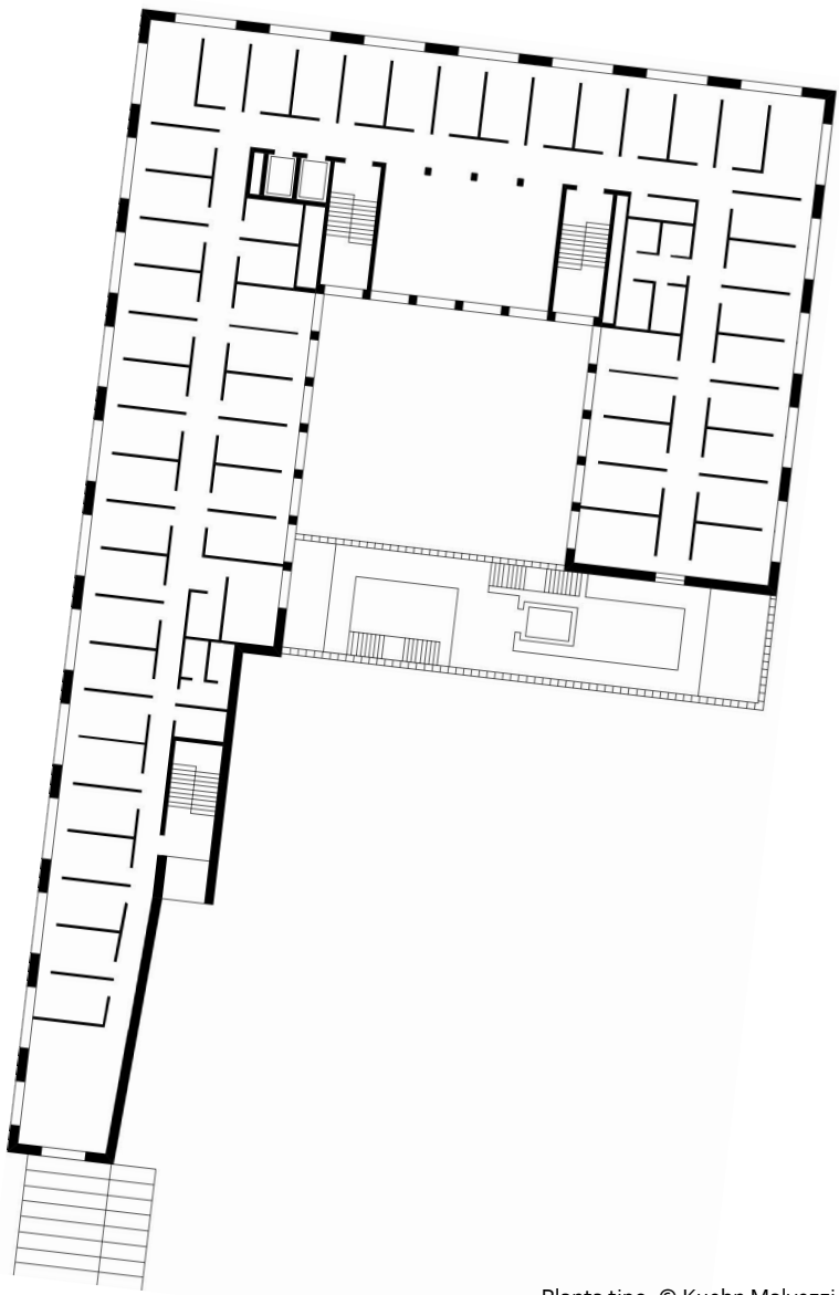
Planta tipo. © Kuehn Malvezzi
