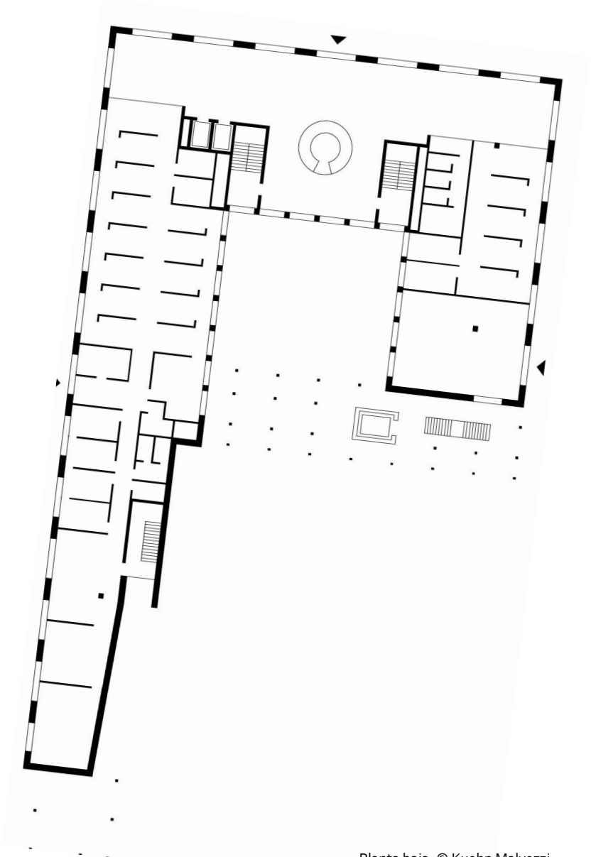
Planta baja. © Kuehn Malvezzi
