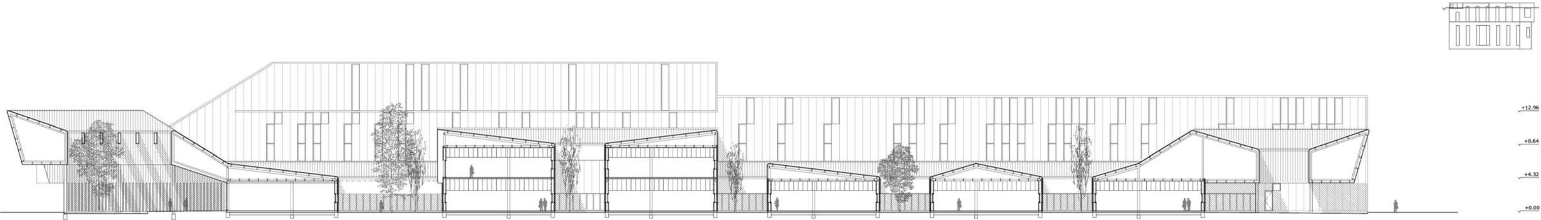
Sección longitudinal. Hospital paramétrico de Manta
