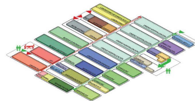
Esquema funcional. Hospital paramétrico de Puyo
