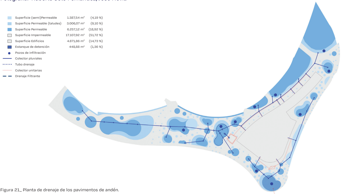
Figura 21_ Planta de drenaje de los pavimentos de andén.
