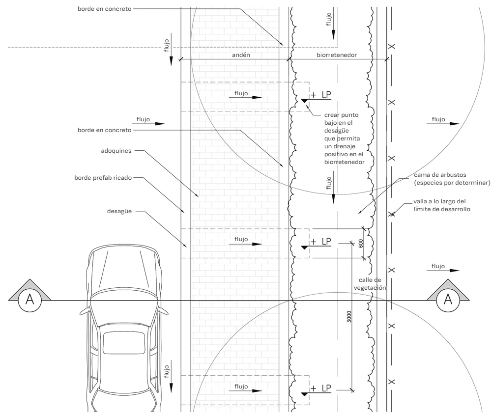
Figura 30_ Planta tipo de biorretenedor de andén
