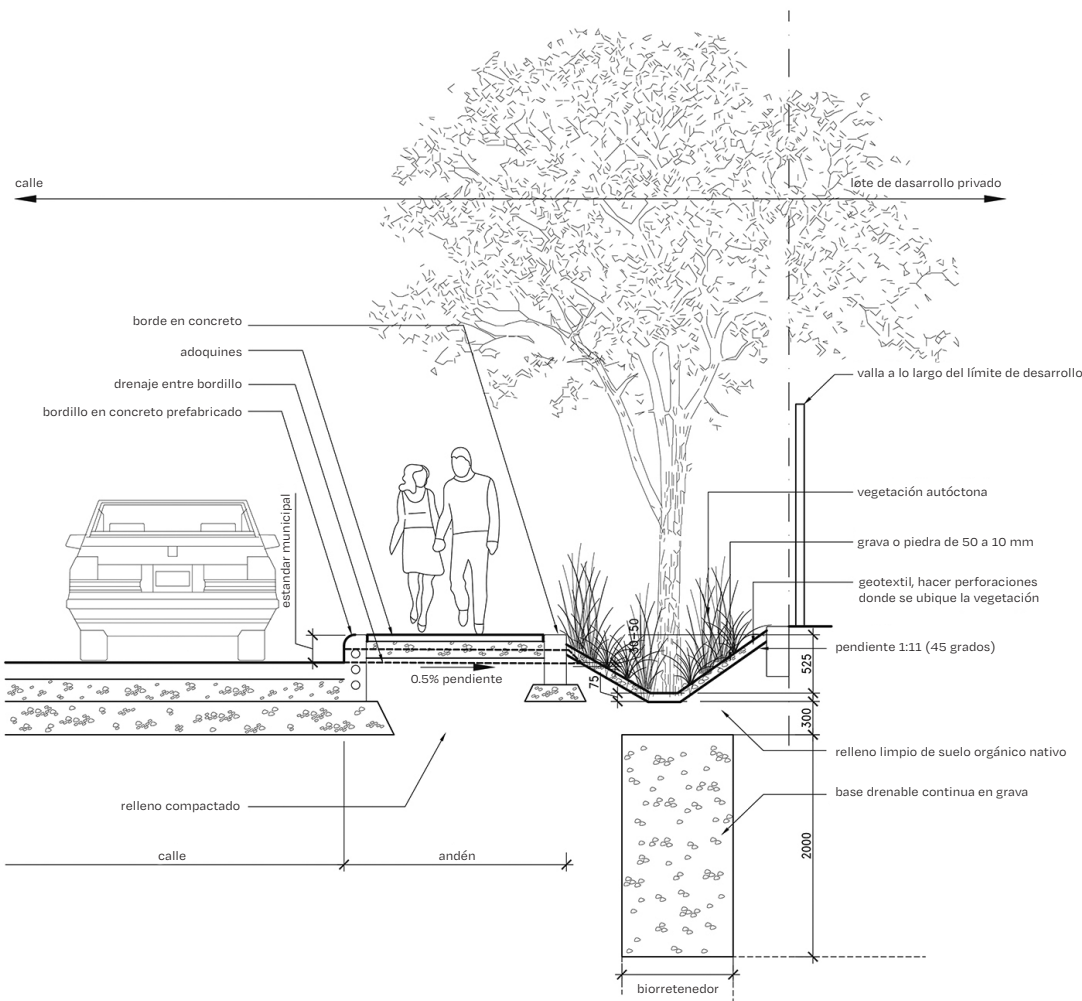
Figura 31_ Sección tipo de biorretenedor de andén
