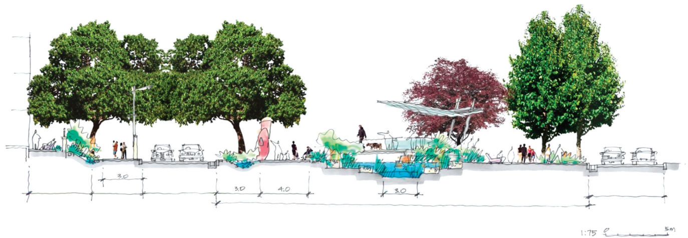
Figura 33_ Corte transversal alameda.
