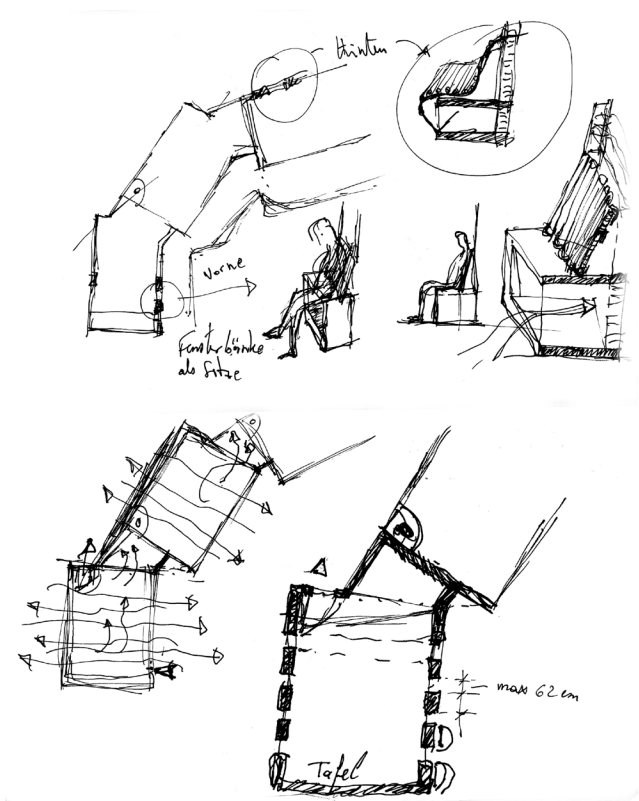
Figura 56_ Dibujo de detalle por Francis Kéré.
