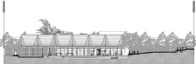
Figura 24_ Conjunto corte transversal.
