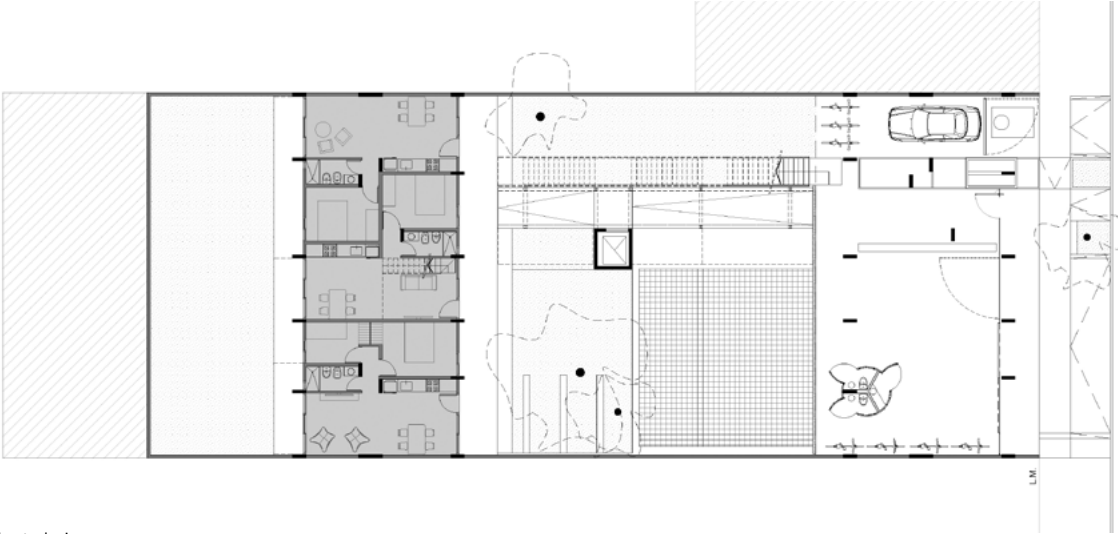
Figura 31_ Planta baja.
