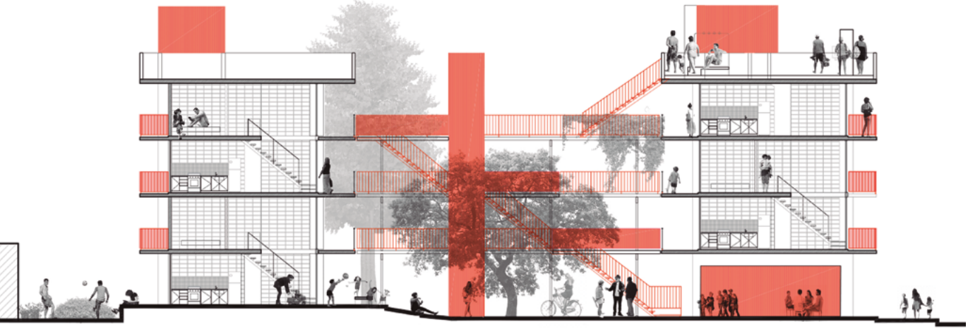
Figura 33_ Corte longitudinal.
